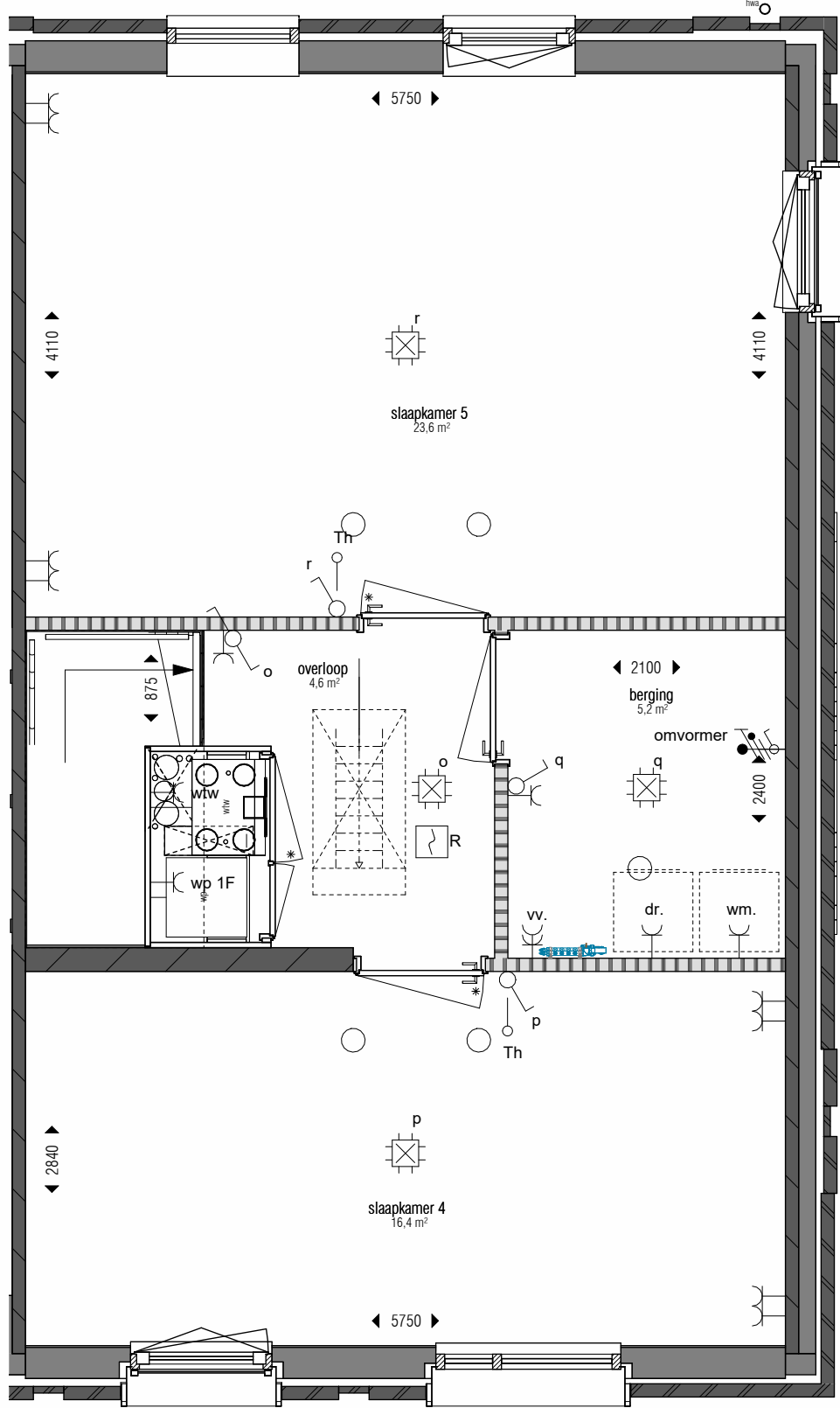
tweede verdieping 1 : 50
