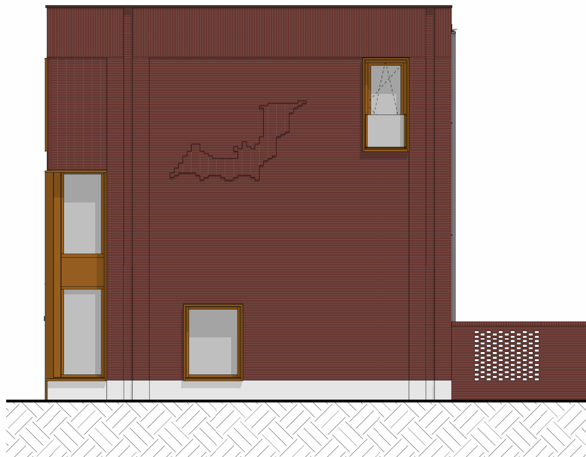
kopgevel 1 : 100
