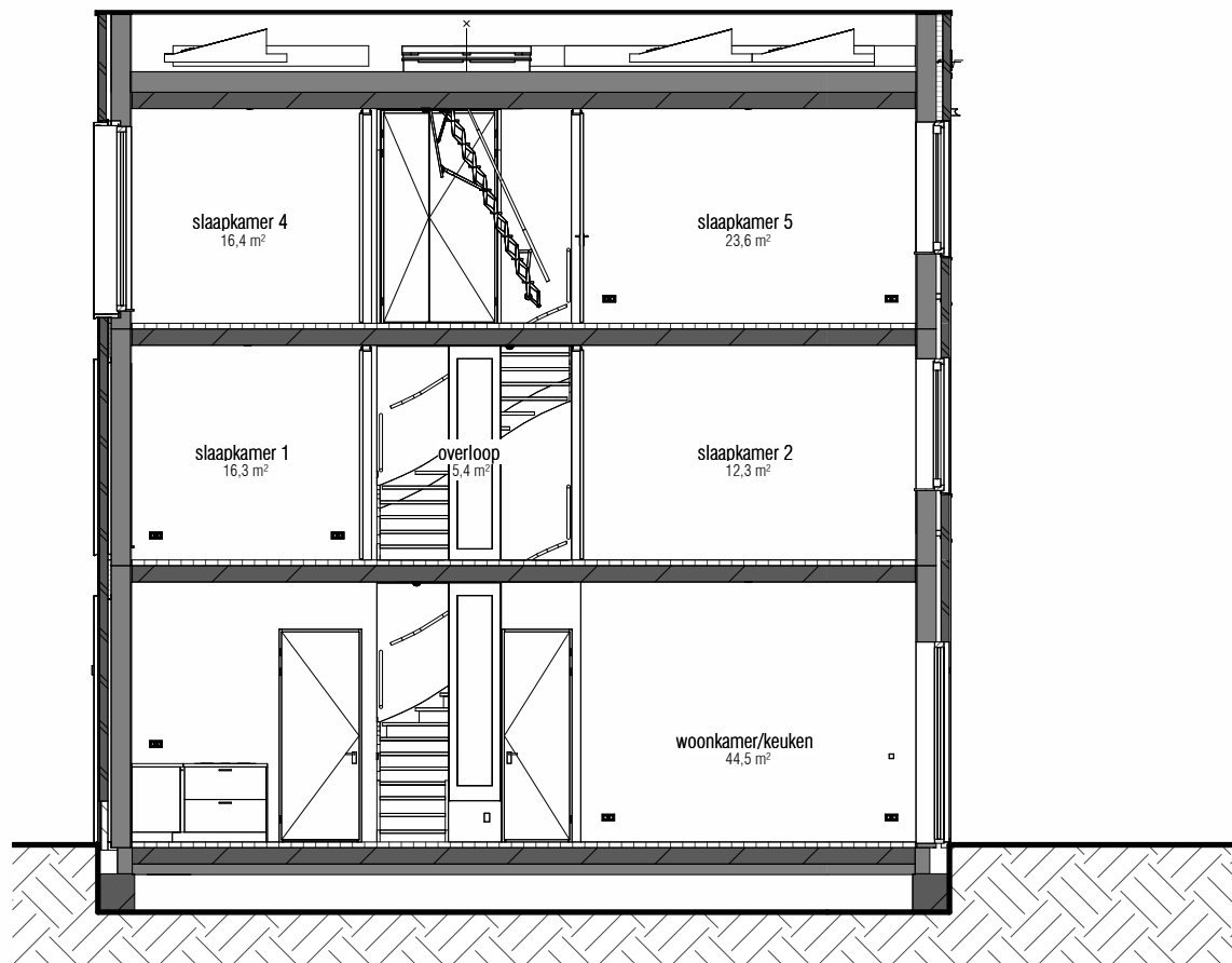
doorsnede 1 : 100
