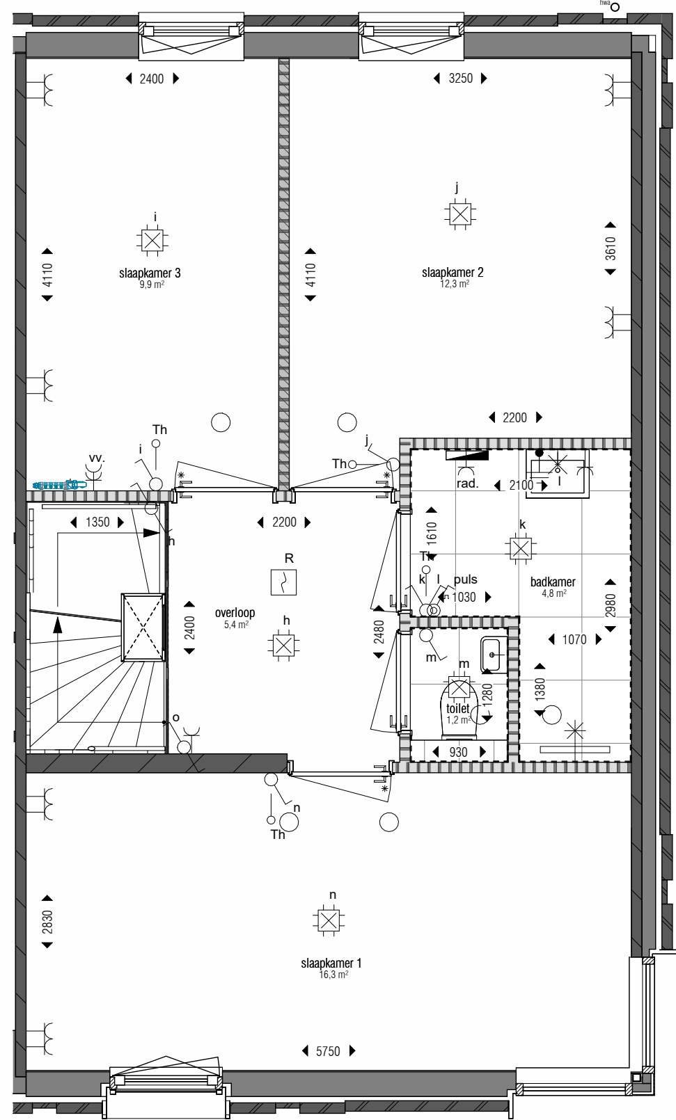
eerste verdieping 1 : 50
