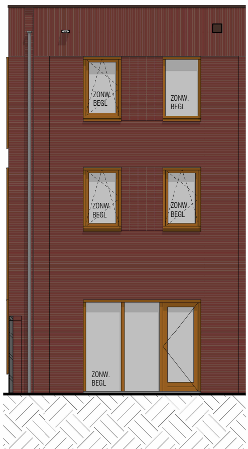
achtergevel 1 : 100
